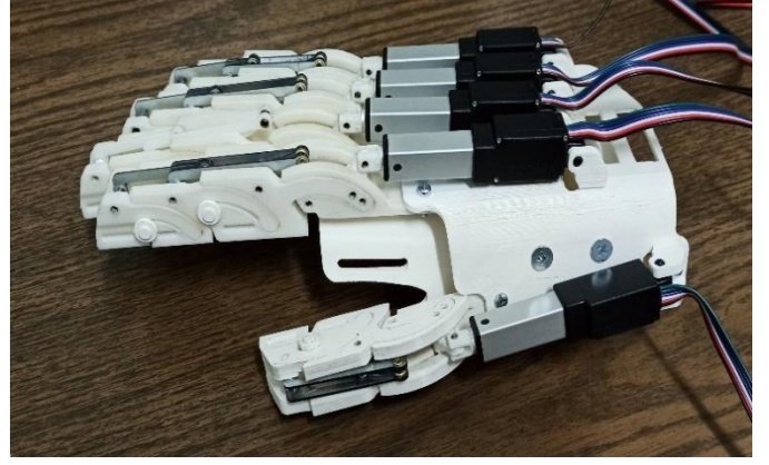
Şekil 2. Çalışma kapsamında tasarımı yapıp üretimi gerçekleştirilen harici el iskelet prototipi
