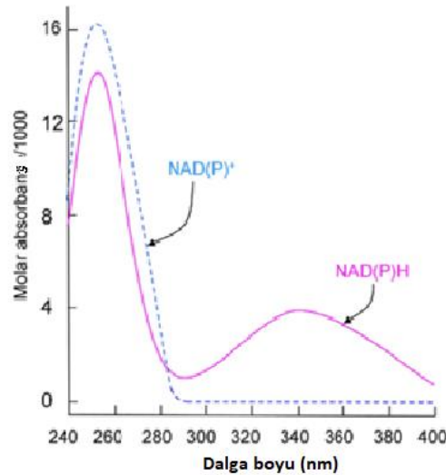
Şekil 2: NAD(P)+ ve NAD(P)H moleküllerinin absorbans spektrumu [5].
