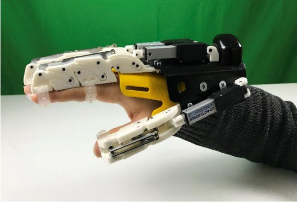
Şekil 2. Çalışma kapsamında tasarımı yapıp üretimi gerçekleştirilen harici el iskelet prototipi
